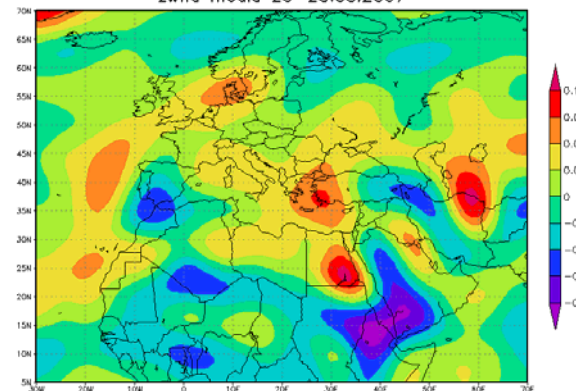
zwnd media 23-28.08.2007
