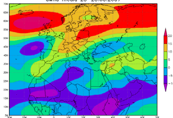
uwnd media 23-28.08.2007
