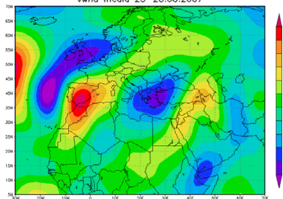
vwnd media 23-28.08.2007
